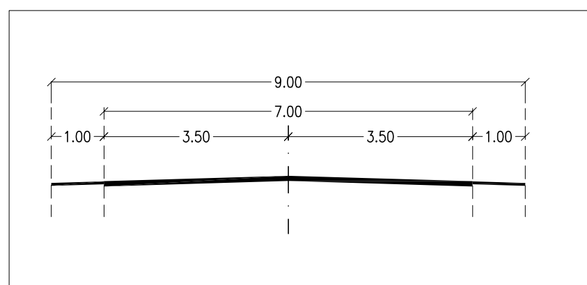
SEZIONE STRADALE TIPO
